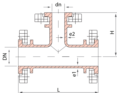
سه راهی سه سر فلنج گردان
