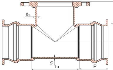
سه راهی دو سر ساکت ناف فلنج جداره نازک Double socket tee with flanged branch-L.Pipe (PE/PVC)
