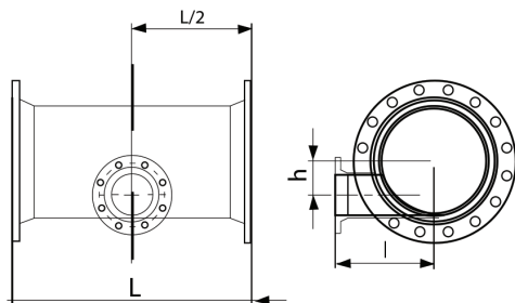
سه راهی سه سر فلنج اینورتنی ‡ All flanged level invert tee
