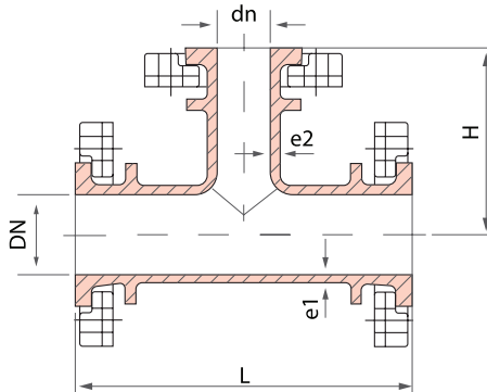
سه راهی سه سر فلنج گردان
