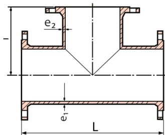
سه راهی سه سر فلنج All Flanged Tee-Series A
