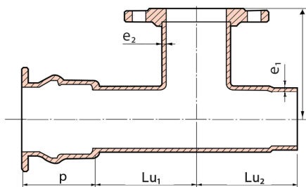
سه راهی ساکت اسپيگات با ناف فلنج جداره نازک Socket-spigot tee with flanged branch-L.Pipe (PE/PVC)
